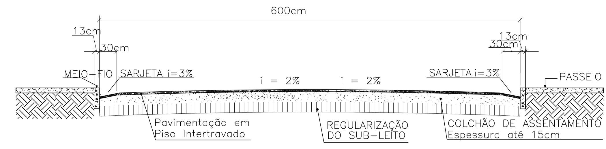
CORTE TRANSVERSAL ESC 1/1
