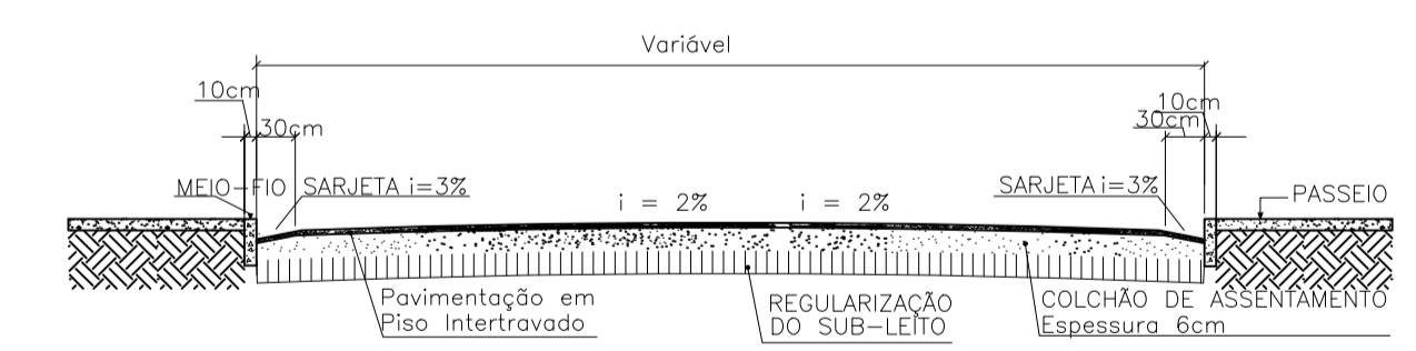
CORTE TRANSVERSAL ESCALA 1/50
